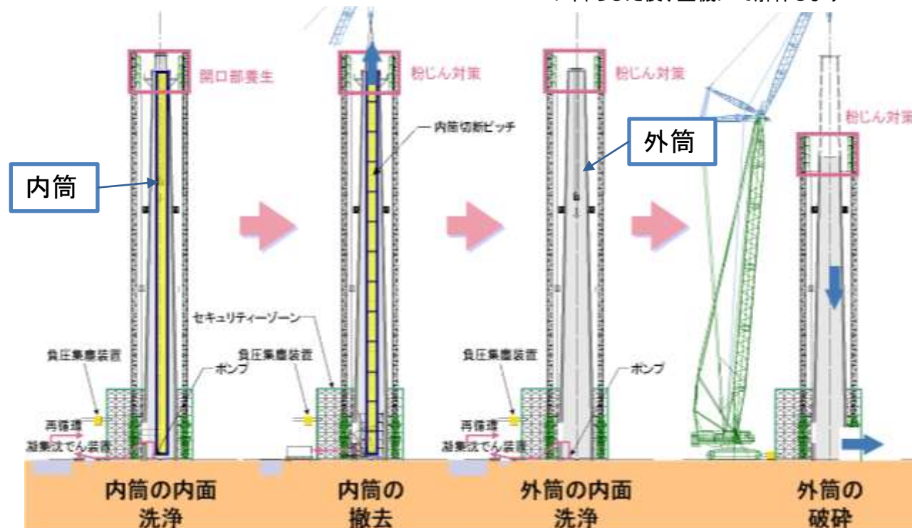
輪切りにしたコンクリートをクレーンで地上に降ろした後、重機にて解体します
