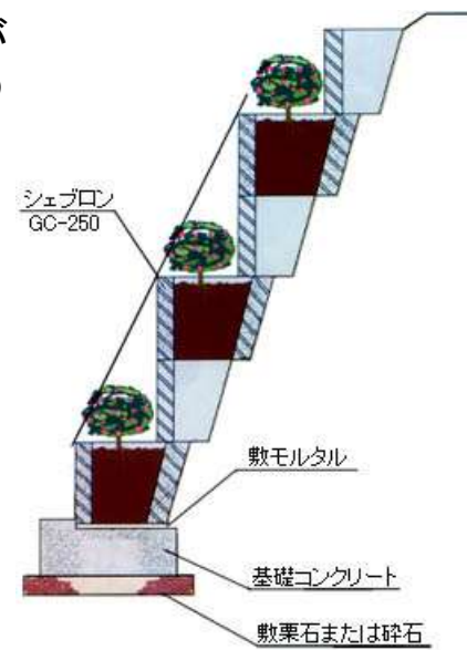
植生ブロック断面図
